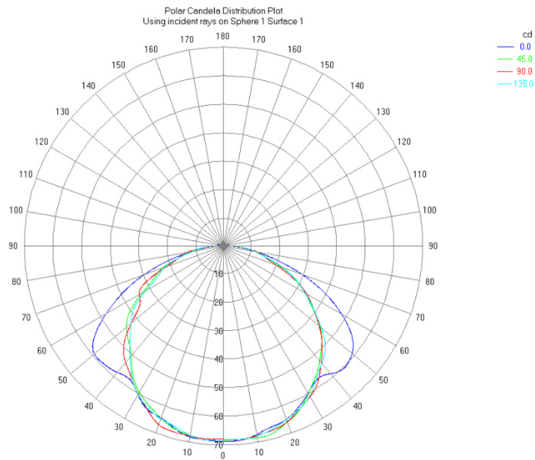
配光曲线图
